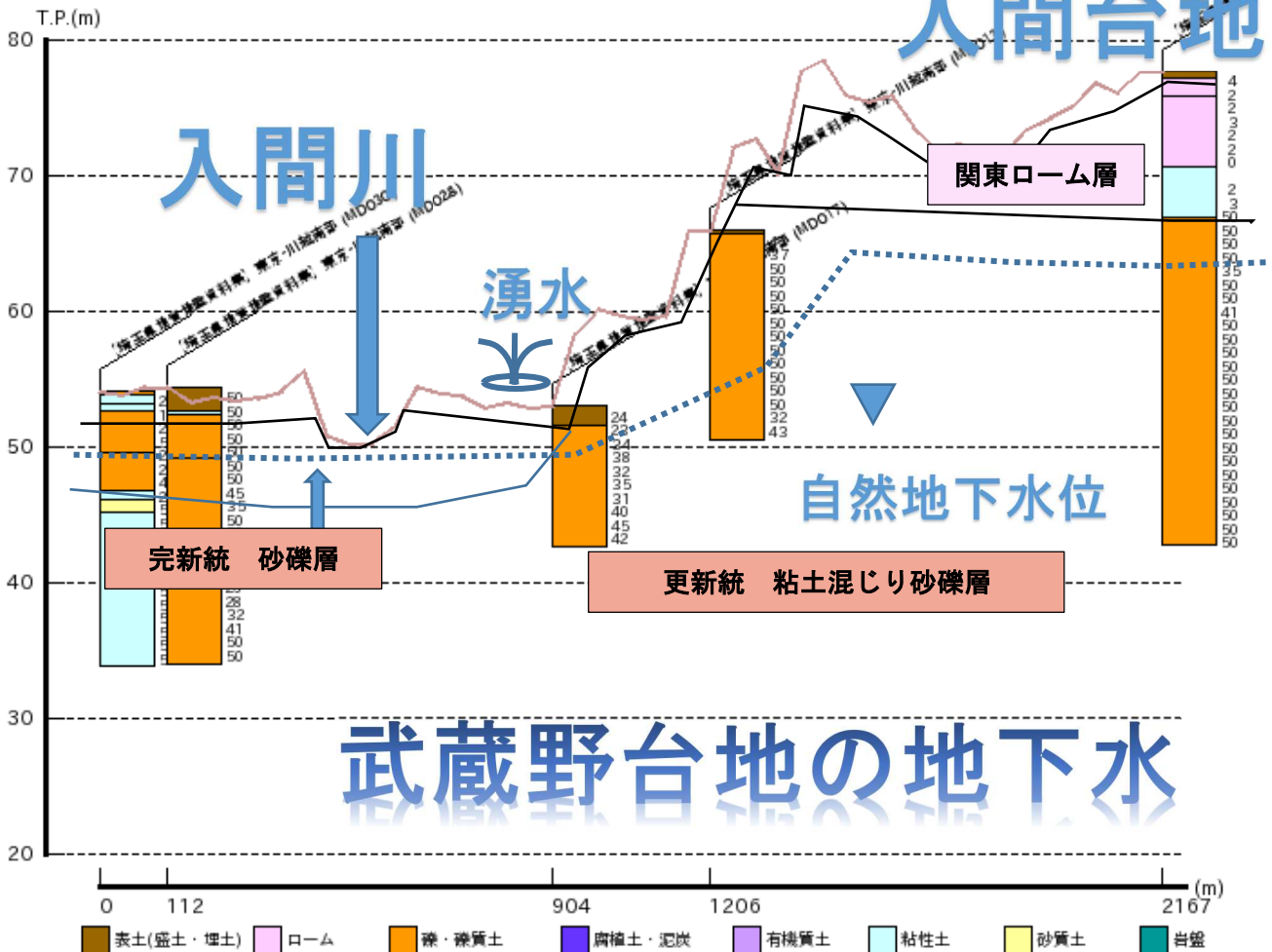
地質断面図
